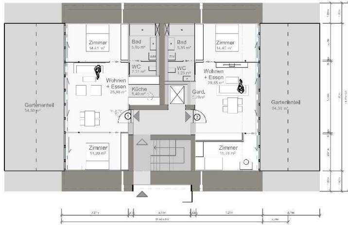
Grundriss EG M 1:100
