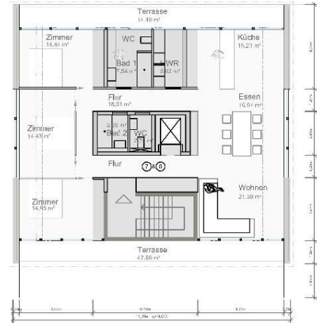
Grundriss OG 4,5 M 1:100
