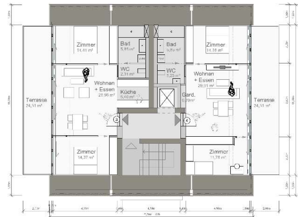
Grundriss 1. OG M 1:100
