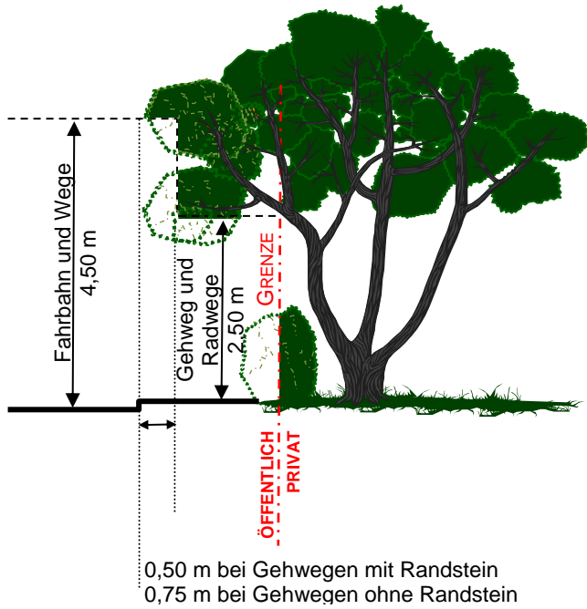
Lichtraumprofil Straße
